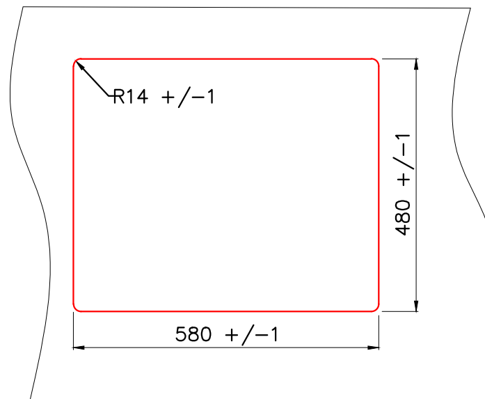
Врезной монтаж мойки (I)
