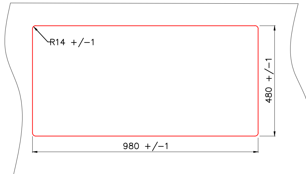
Врезной монтаж мойки (I)
