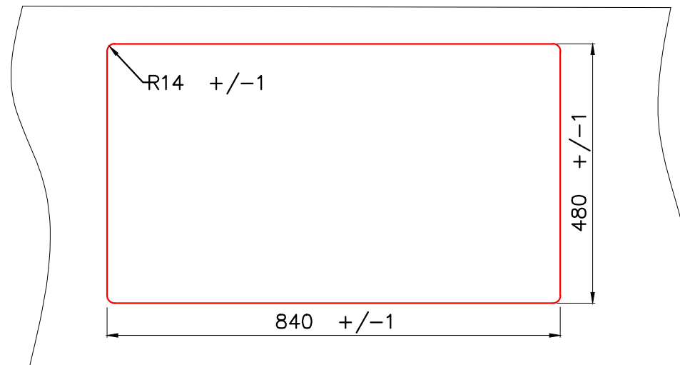
Врезной монтаж мойки (I)
