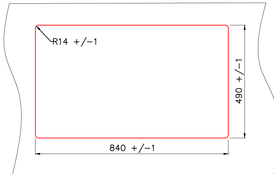
Врезной монтаж мойки (I)
